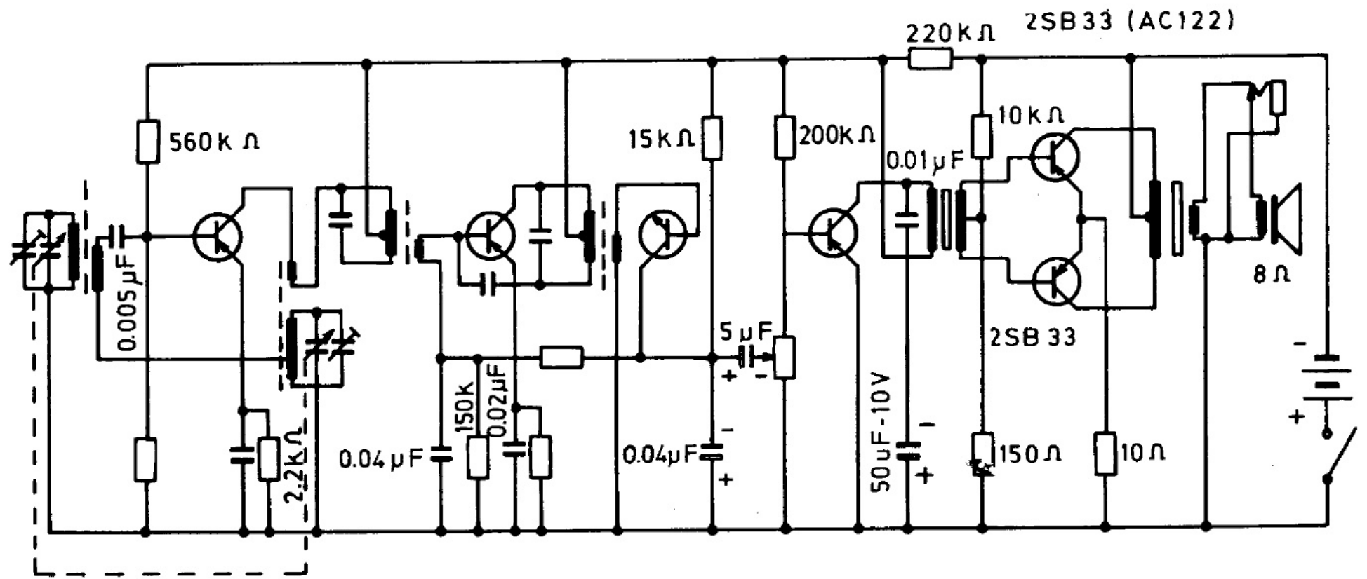
SCHEMA ELETTRICO DEL RADIORICEVITORE G.B.C. AR/12B
